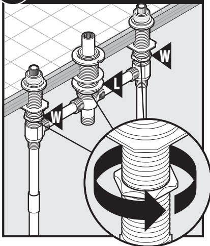
B8 Finished Deck / Cubierta terminada / Plate-forme finie
