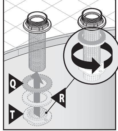
B11 Finished Deck / Cubierta terminada / Plate-forme finie
