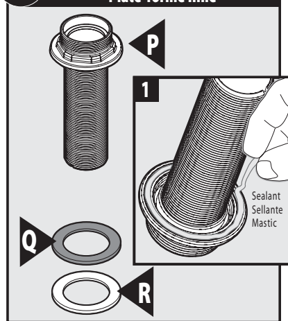
B9 Finished Deck / Cubierta terminada / Plate-forme finie
