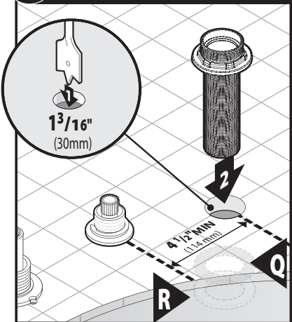
B10 Finished Deck / Cubierta terminada / Plate-forme finie
